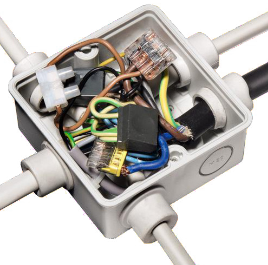
conventionele verdeeldoos
